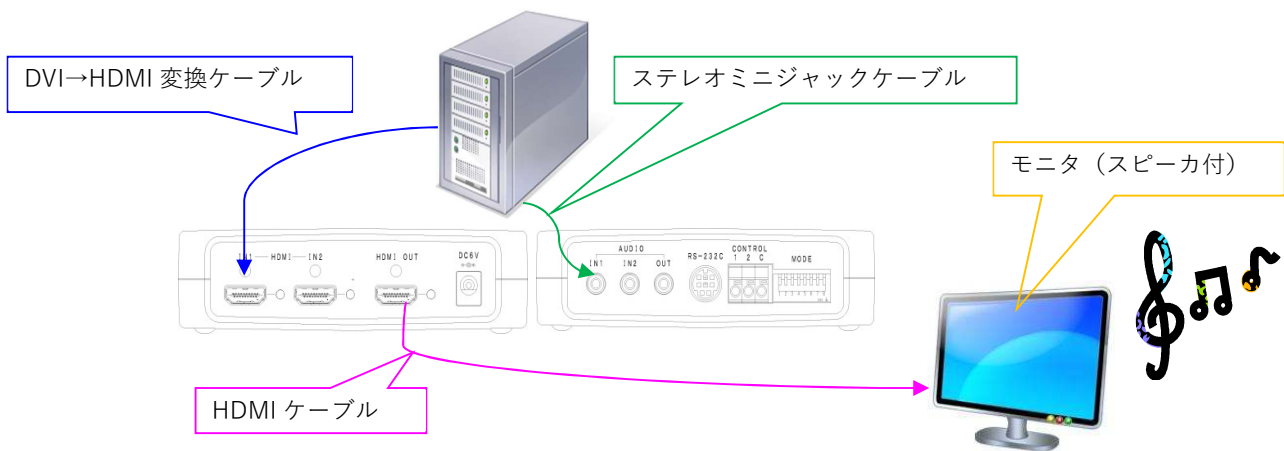
図 2 DVI 出力/アナログ音声出力の PC を HDMI モニタ（スピーカ内蔵）に接続した場合
