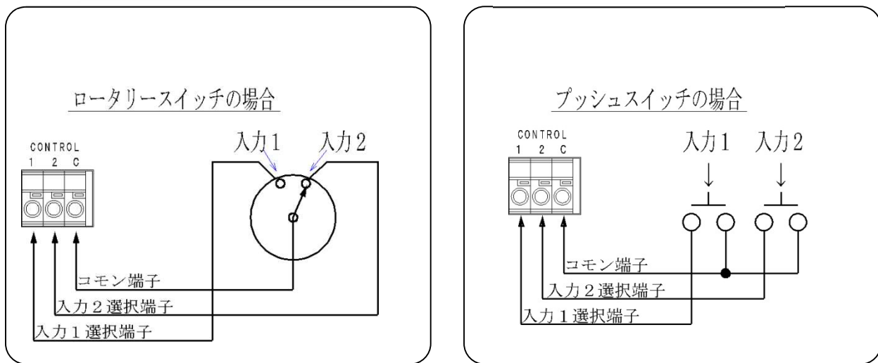
図 5 外部コントロール端子接続例
