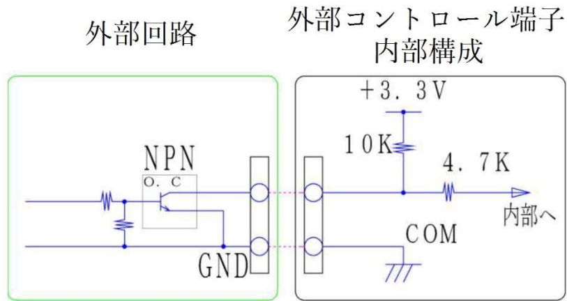
図 6 電子制御参照回路
