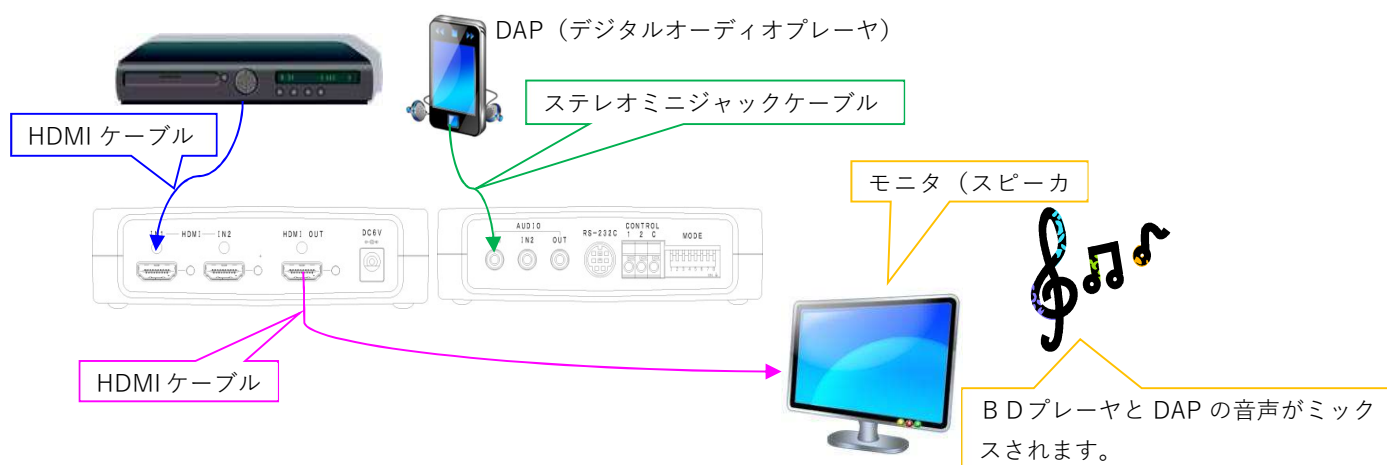
図 3 HDMI 出力とアナログ音声出力を接続して HDMI モニタに接続した場合
